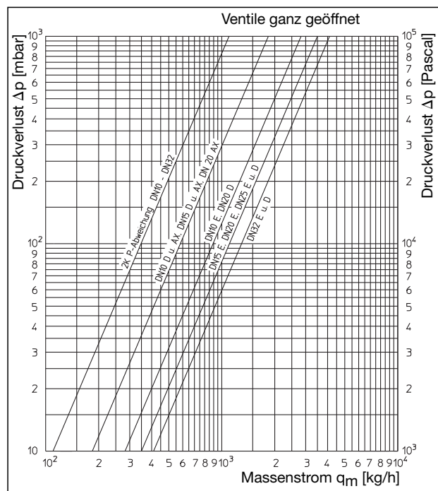
Leistungsdaten Diagramm 2
