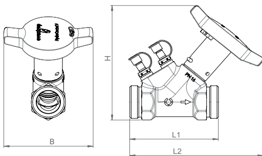
Fig. 3: Mått sidovy / frontvy yttergånga
