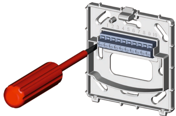
Abb. 9: ClimaCon F elektrisch anschließen
