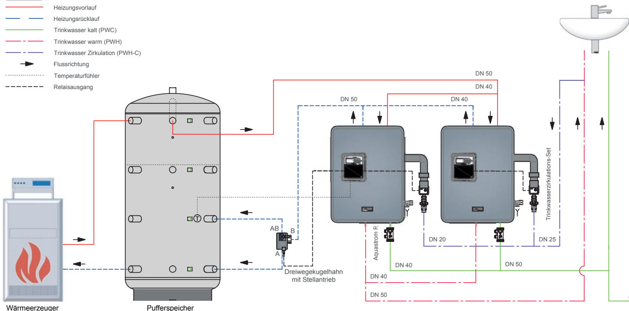
Abb. 3.6: Anlagenschema mit zwei Frischwasser-Stationen „Regumaq X-80“ („Tichelmann-System“)
