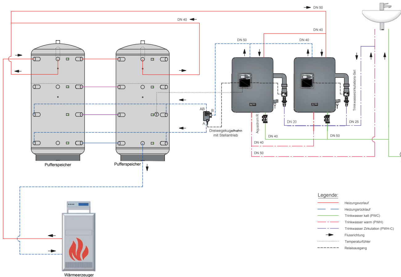
Abb. 3.7: Anlagenschema mit zwei Pufferspeichern und zwei Frischwasser-Stationen („Tichelmann-System“)
