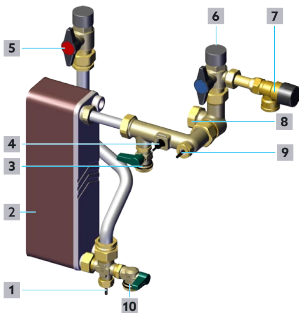
Abb. 31: Trinkwasserkreis
