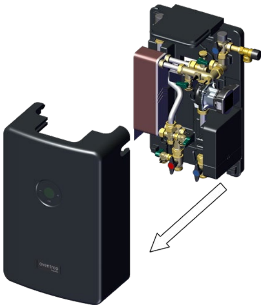
Abb. 10: Oberschale abnehmen
