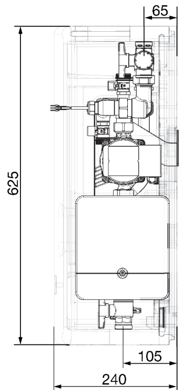
Dimensiuni Regumaq X-25 (vedere laterală)
