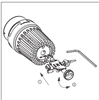
Temperatureinstellung Thermostat „Uni LHB“ Temperature setting thermostat “Uni LHB” Réglage de la température thermostat «Uni LHB»
