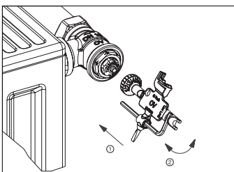
Voreinstellung Ventile „Baureihe AV 9“ Presetting valves “Series AV 9” Préréglage robinets «Série AV 9»
