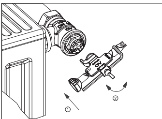
Voreinstellung „Q-Tech“ (z.B. Ventile „Baureihe AQ“) Presetting “Q-Tech” (e.g. valves “Series AQ”) Préréglage «Q-Tech» (par ex. robinets «Série AQ»)
