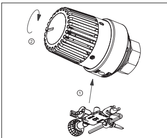
Demontage Handgriff Thermostat „Uni LH“ Removal handgrip thermostat “Uni LH” Démontage poignée manuelle thermostat «Uni LH»
