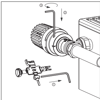
Montage/Demontage „Uni LHB“ Installation/removal “Uni LHB” Montage/démontage «Uni LHB»
