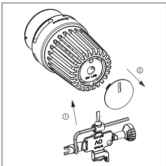
Demontage der Abdeckscheibe Thermostat „Uni LHB“ Removal of the cover disc thermostat “Uni LHB” Démontage du capot thermostat «Uni LHB»
