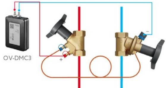
图 7: 连接图 OV-DMC3
