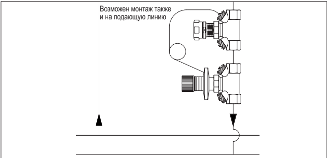
Пример: Регулирование расхода с помощью регулятора перепада давления „Hysocop DP“ и регулирующего вентиля „Hysocop V“.
