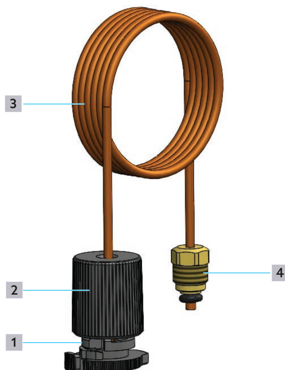
Ryc. 4: Budowa przewodu impulsowego
