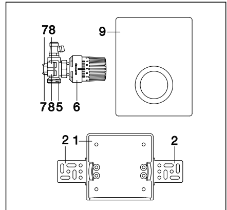
Komponenten Umrüstsatz
