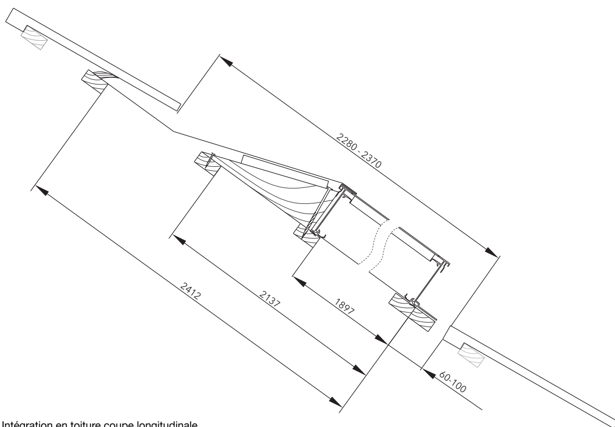
Intégration en toiture coupe longitudinale
