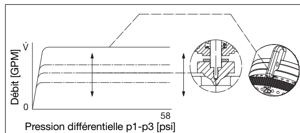
Fig. 5.5 Ligne caractéristique du débit pour pré-réglages différents
