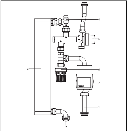
Abb. 31 Primärkreislauf
