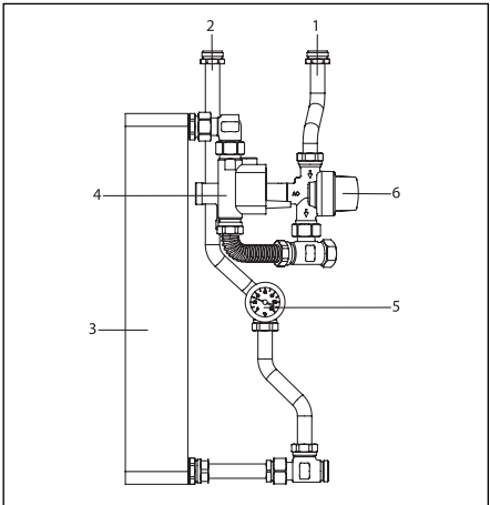
Abb. 32 Sekundärkreislauf
