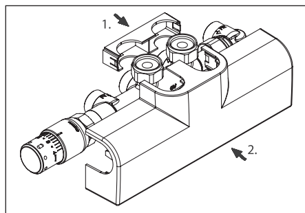
Abb. 13 Montage Design-Abdeckung
