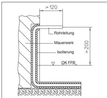
Abb. 7 Schnitt, Heizkreisanschluss
