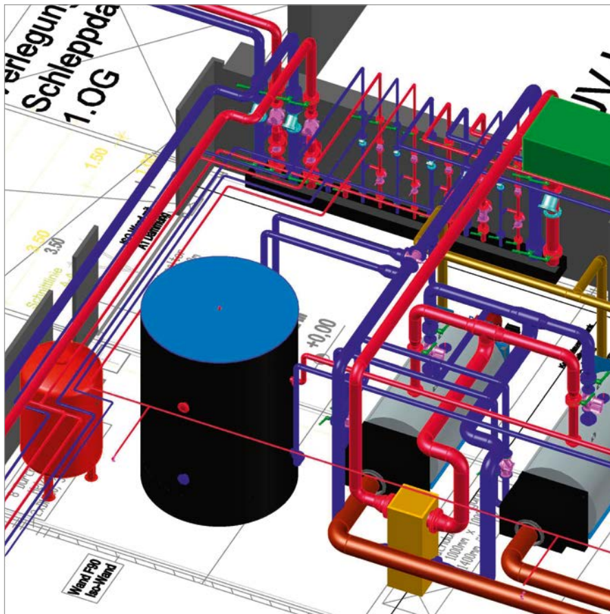
Diseño con "BIM": Ejemplo de una calefacción central con productos Oventrop
