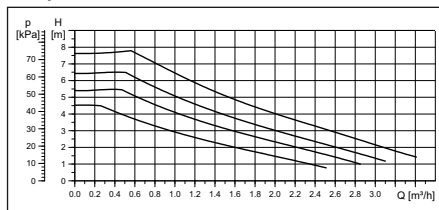
Abb. 5.4 Pumpenkennlinie Grundfos UPM 3
