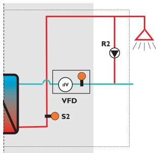
Circuito secundario
