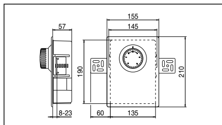
Encombrements
