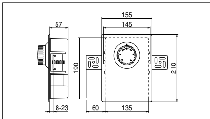
Maße
