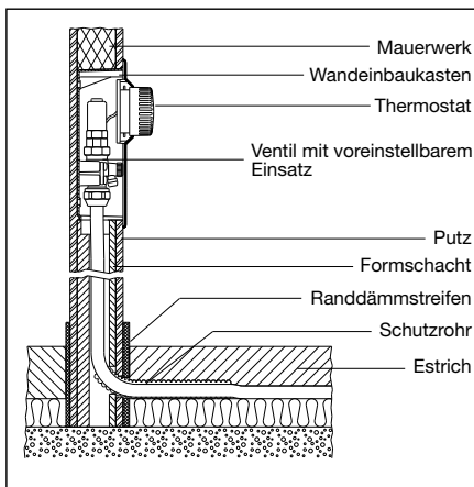
Schnitt
