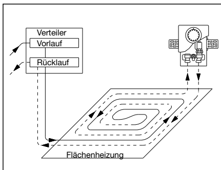
Einbauskizze
