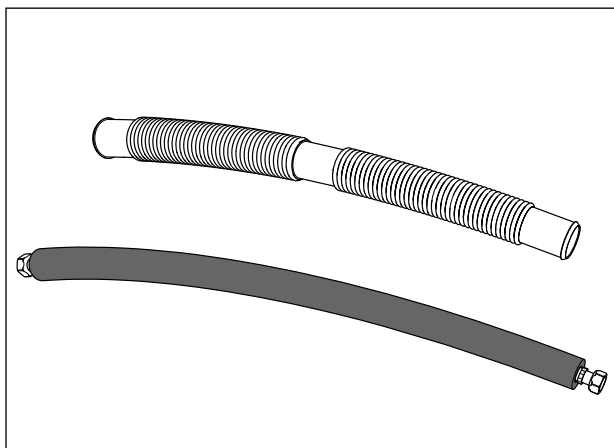
Abb. 1 Kollektorschlauchanschluss: Edelstahlwellenschlauch mit Isolierung und UV-beständigem Faltenbalg gegen Tierverbiß.
