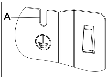
Abb. 7.1 Schutzpotentialausgleich/Erddung
