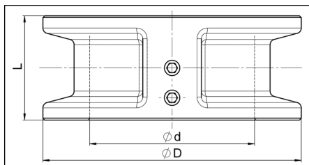
Fig. 4.1 Dimensions du clapet de retenue à battant double
