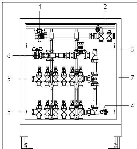
Abb. 5.1: Übersicht Rücklaufsammler
