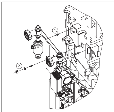
Abb. 17 Montage Solargruppe
