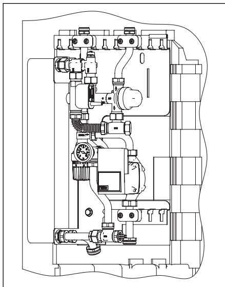
Abb. 13 Montage Frischwasserstation
