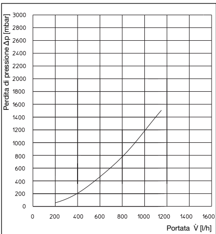
Perdita di pressione circuito secondario (acqua sanitaria) per funzionamento a ricircolo
