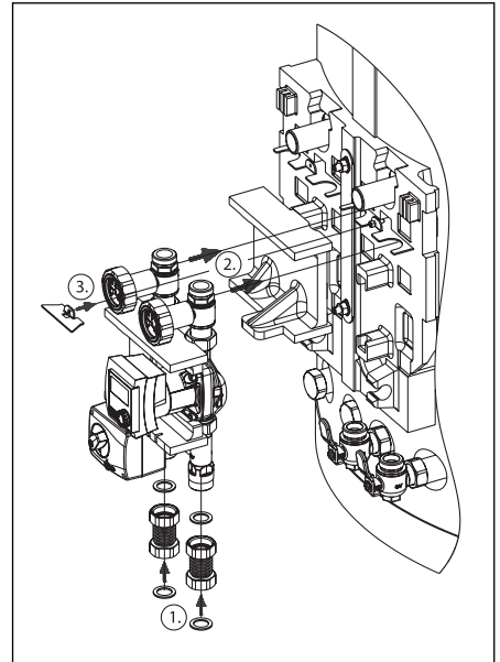
Abb. 10 Montage Heizkreisgruppe
