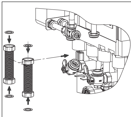
Abb. 14 Montage Metallwellrohre
