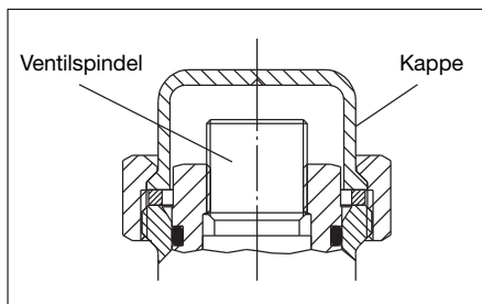
Abb. 7.1: Regulierventil
