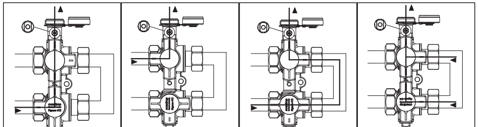
Entleeren der Anlagenseite und Geräteseite Draining of system and appliance side, bleeding and flushing the system side Vidange du côté installation et appareil, purge et rinçage du côté installation
