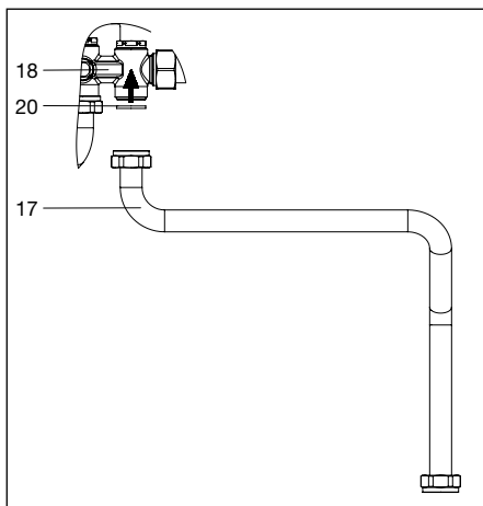
Abb. 6.2 Montage
