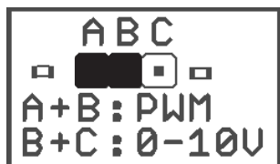
Position du cavalier pour le signal PWM
