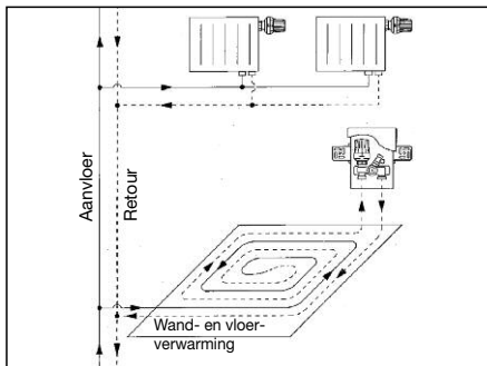
Inbouwtekening
