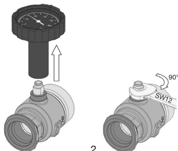
Abb. 21: Pumpenkugelhahn absperren
