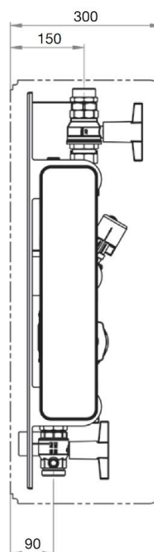
Encombremments Regumaq X-70 (vue de côté)
