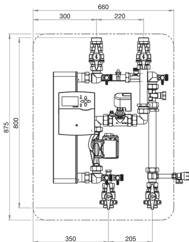
Encombremments Regumaq X-70 (vue de face)
