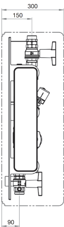
Dimensiones Regumaq X-70 (lateral)
