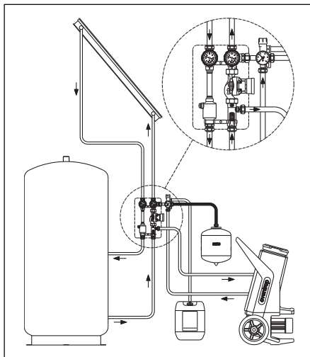
Obr. 6.14 Naplnění pomocí bezpečnostní soupravy a průtokoměr
