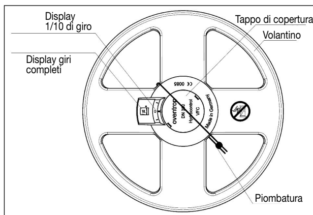
Fig. 7.1 Preregolazione
