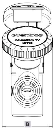
Fig. 3: Dimensiones frontales
