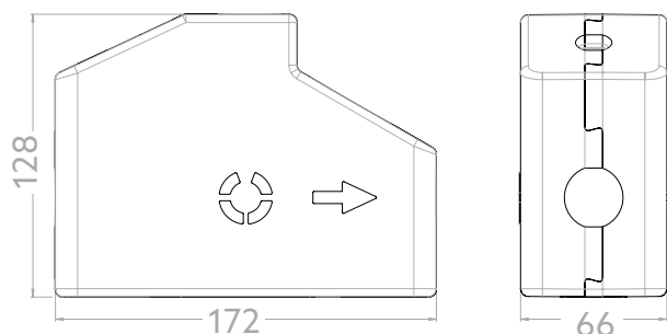
Ryc. 5: Powłoka izolacyjna
