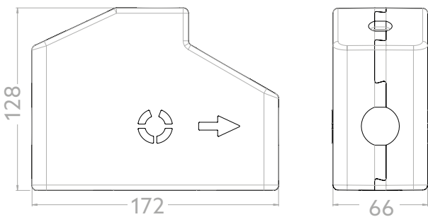
图 5： 绝缘壳
