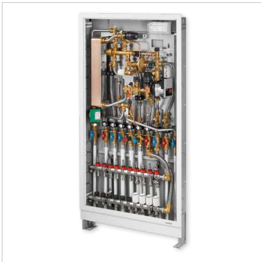
Regudis W-HTF, compleet
