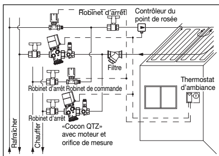
6.2 Système à quatre tuyaux
