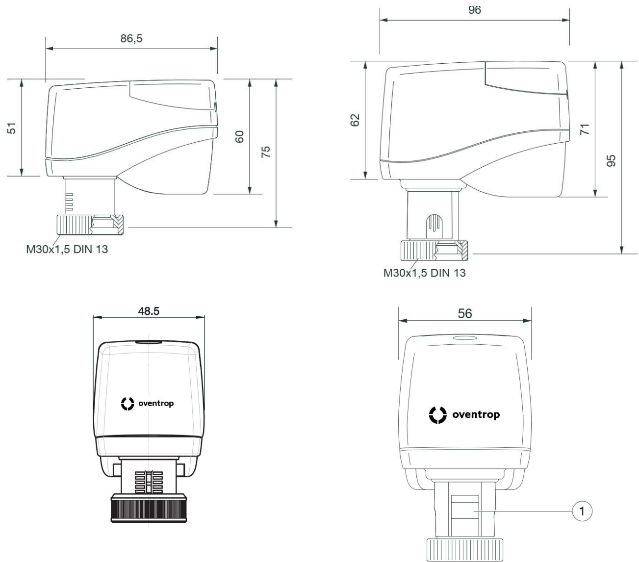
(1) Bouton-presseur pour libérer la tige de la vanne enclenchée
