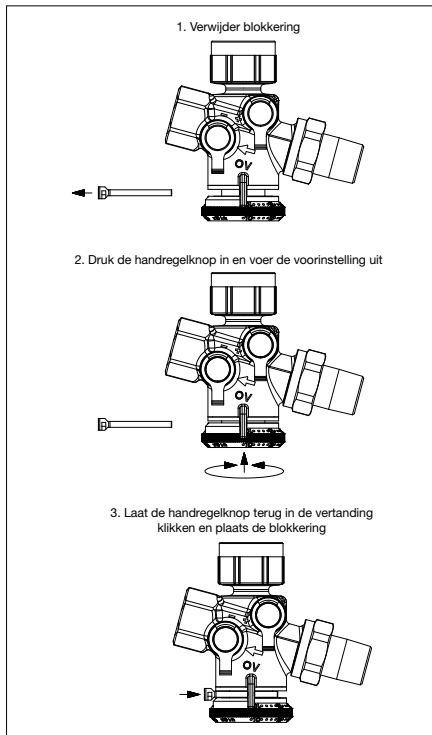
Afb. 7 Debietinstelling
