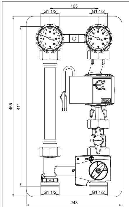
Abb. 4 „Regumat M3-180“ DN25 mit Pumpenkugelhahn (lange Bauform)
