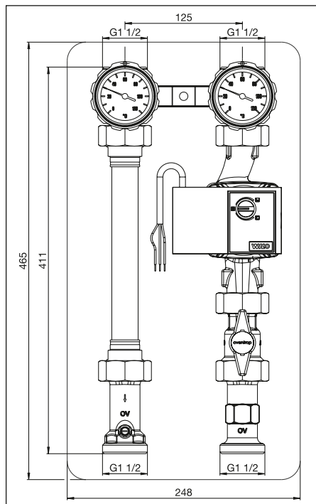
Fig. 3 «Regumat S-180» DN 25 avec robinet d'isolement à tournant sphérique (forme longue)
