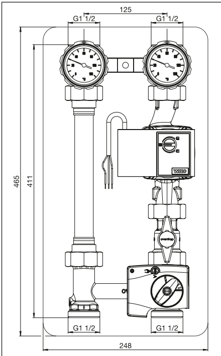
Fig.4 “Regumat M3-180” DN25 con valvola a sfera prima del circolatore (versione lunga)
