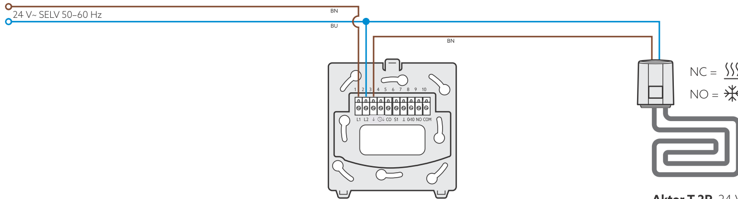
Aktor T 2P 24 V Elektrothermischer Stellantrieb Electrothermal actuator
