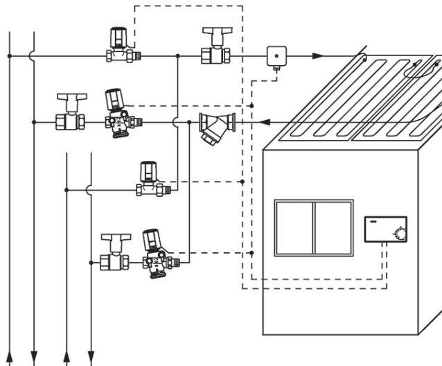
Abb. 7: Einbaubeispiel 2: Vierleitersystem
