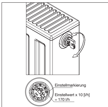
Abb. 4 Durchflusseinstellung
