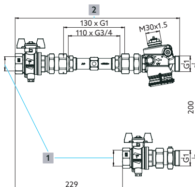
Abb. 4: Abmessungen Durchgangsausführung
