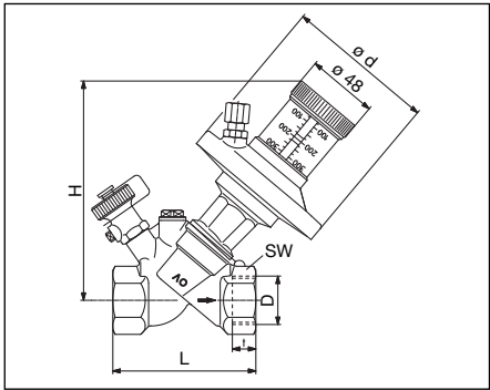
Illustr. 2: Régulateur 10645/4704-16 et 1664706-16 filetage femelle selon EN 10226 des deux côtés
