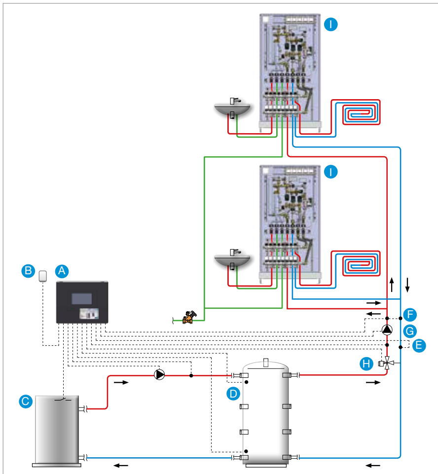
Systeem opbouw
