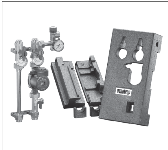
„Regusol”-overgangstation
