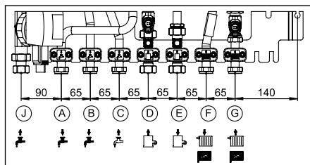
Fig. 4.4 Cotes de raccordement
